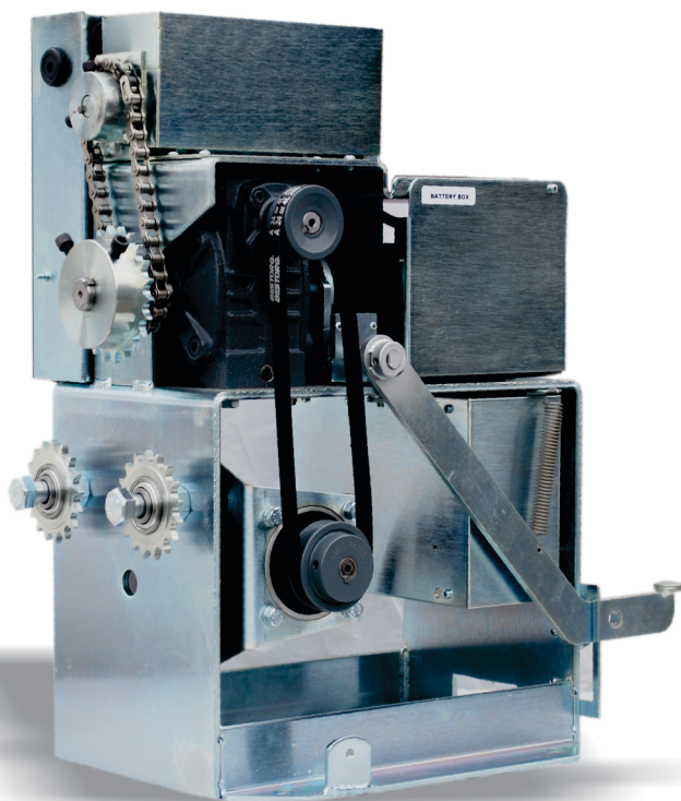
SL-100DCFP
